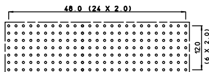
LAY-OUT P.C.B. - HOLE
