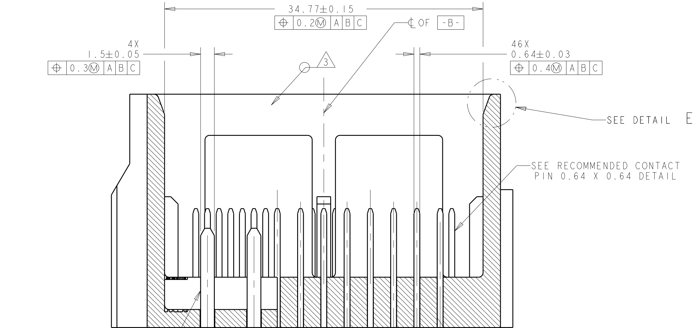
SECTION A-A
