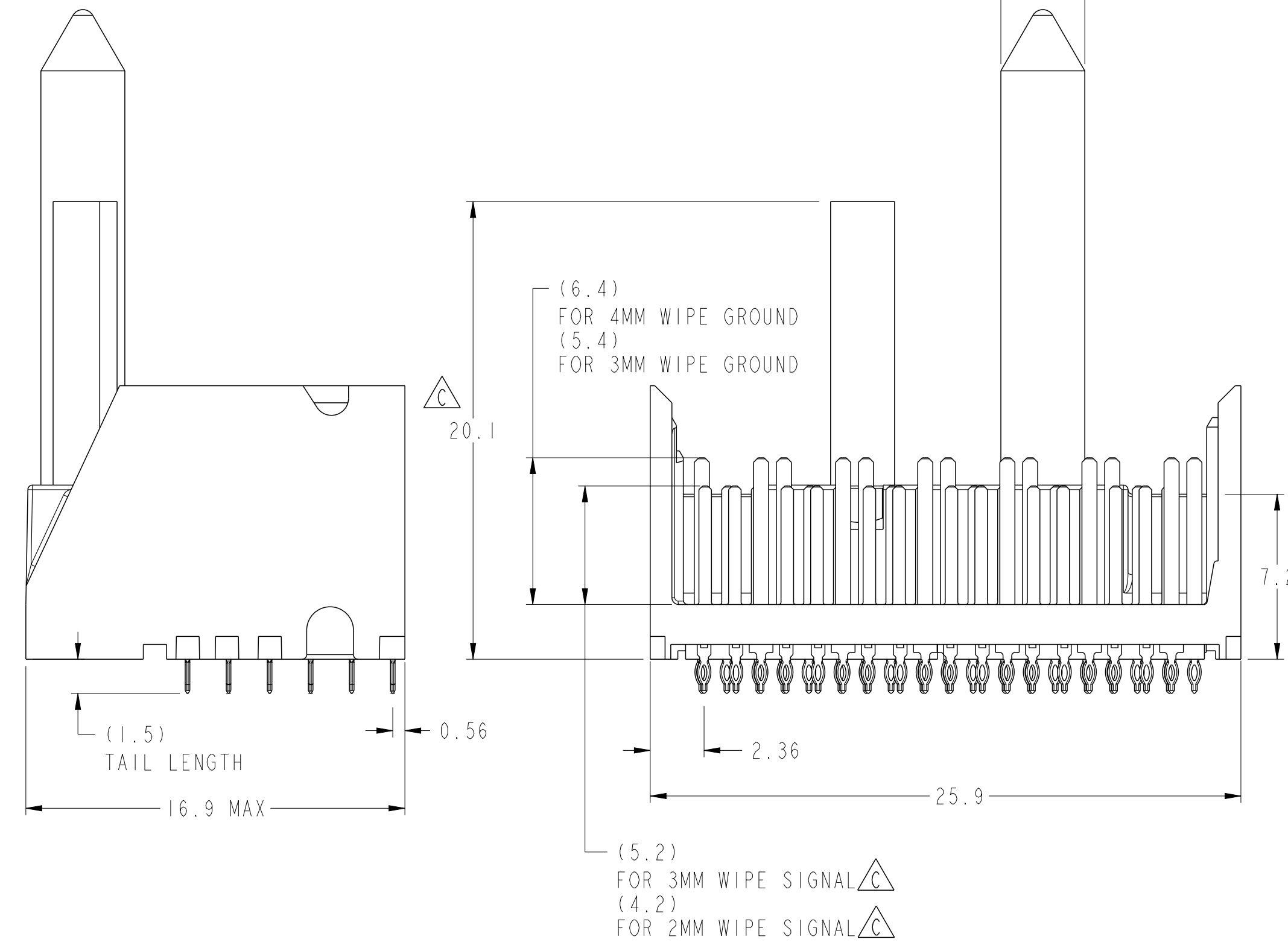
RIGHT POLARIZING GUIDE MODULE
