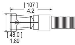
Thread Conduit Adapter
