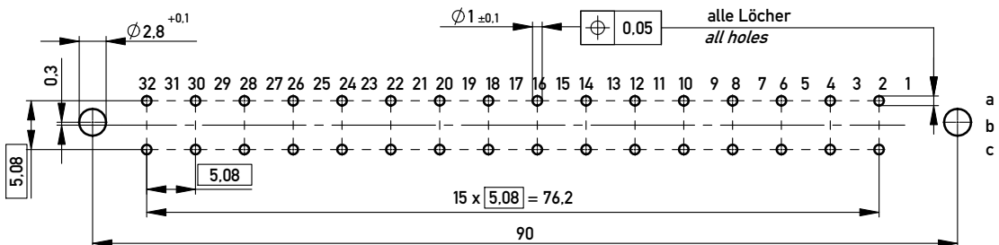
Leiterplatten-Lochbild / PCB drillhole pattern
