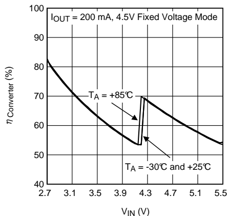
4.5-V Mode
