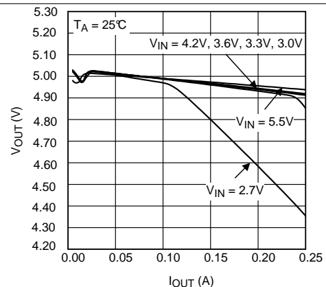
5-V Mode
