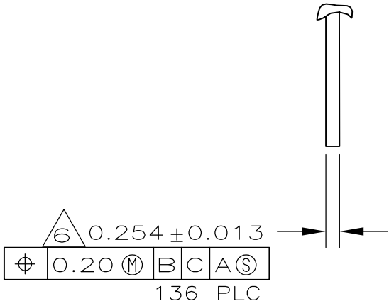
DETAIL Y SCALE 1 O: 1
