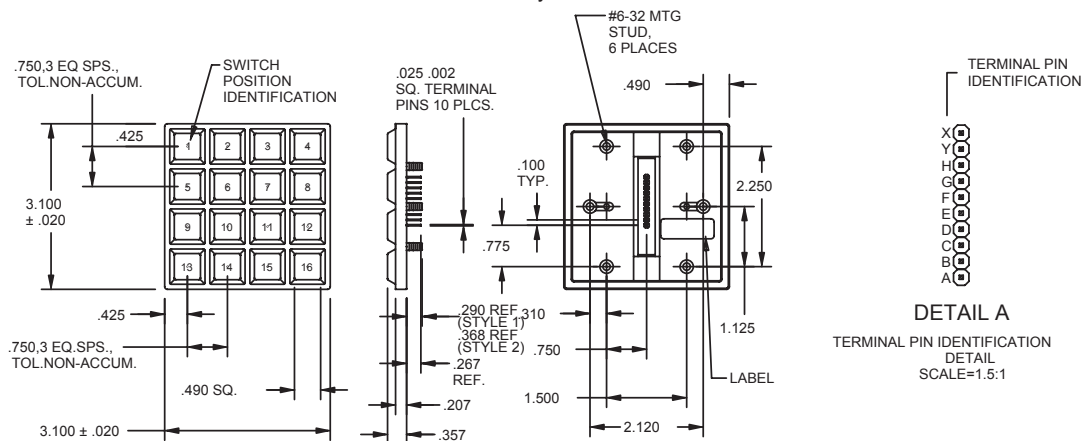
4 x 4 Keyboard
