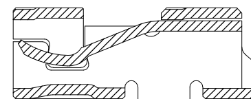
A-A (P/N1827395-1)
