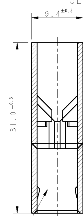
SEZIONE A-A SECTION A-A
