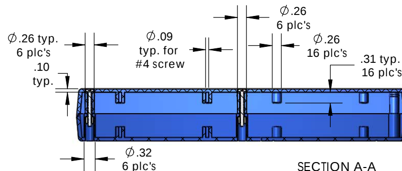
SECTION A-A SCALE 1 : 2.75
