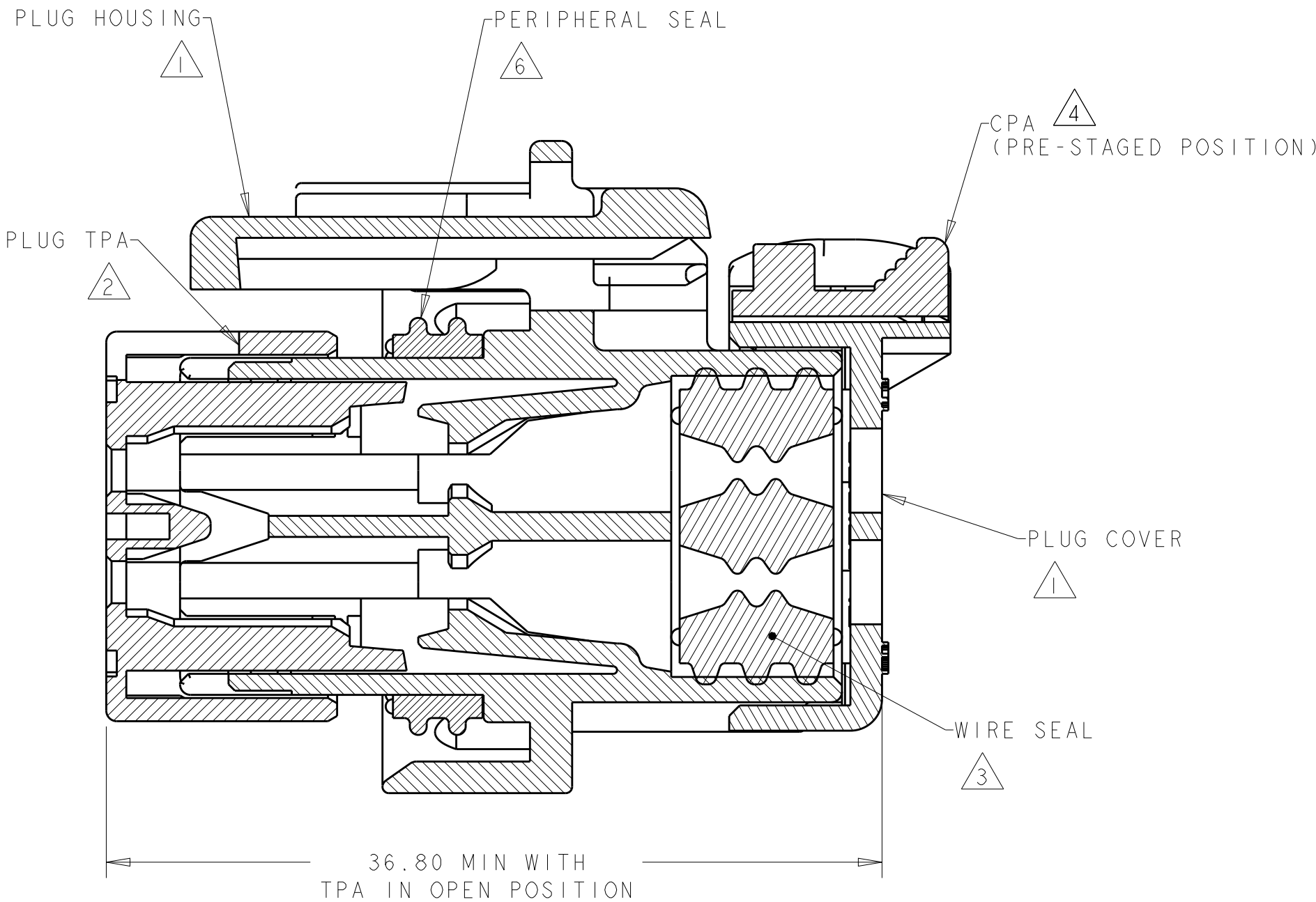
SECTION A-A
