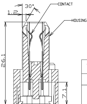
SECT A-A
