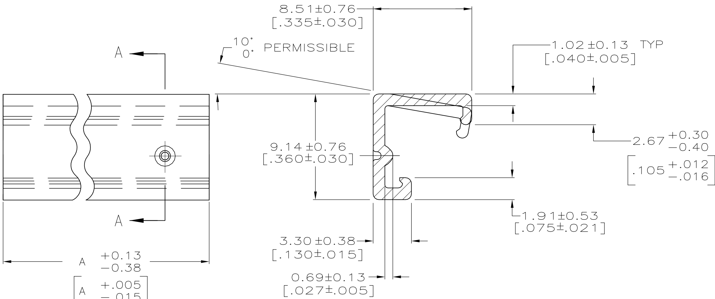
SECTION A-A
