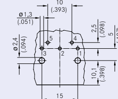
5 POL S 1)
