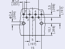
7 POL 1)
