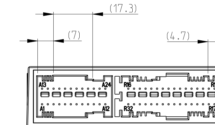
0-1418939-9 AC-Ac / RA_Ra-RI_R
