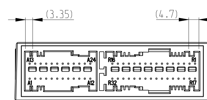
0-1418939-4 AB-Ab / RA_Ra-RI_R
