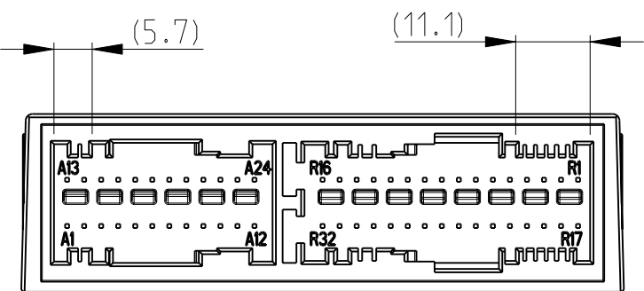
AA-Aa 0-1418939-3 / RE_Re-RI_Ri
