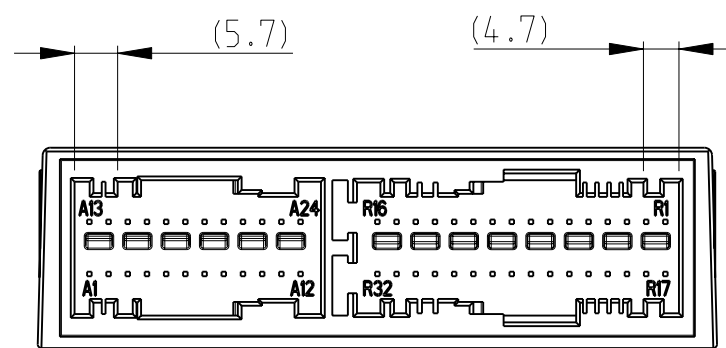
AA-Aa 0-1418939-1 RA_Ra-RI_RI
