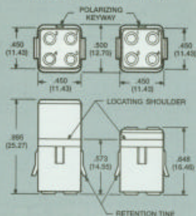
Socket Module LMD-3005-S
