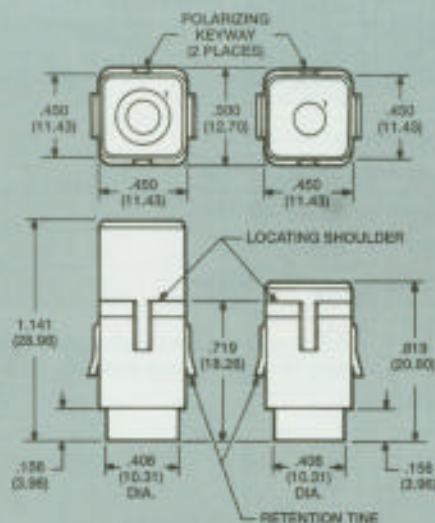
Socket Module LMD-3004-S
