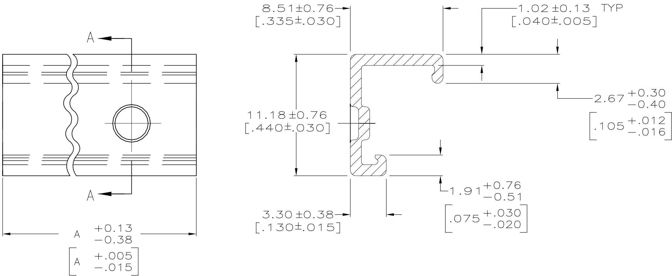
SECTION A-A
