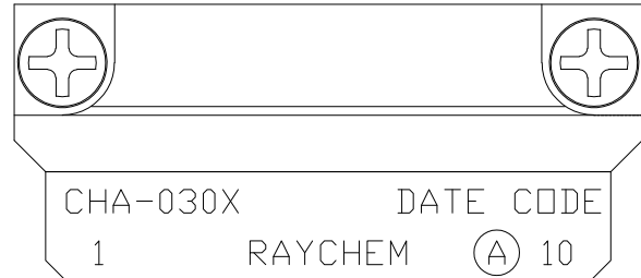
RECEPTACLE
