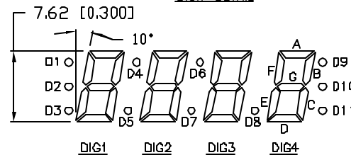
DIGIT DETAIL
