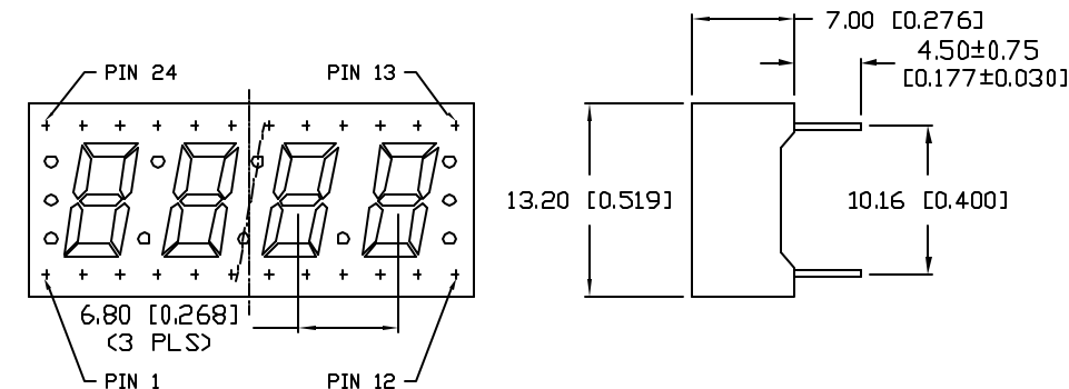
DIGIT DETAIL
