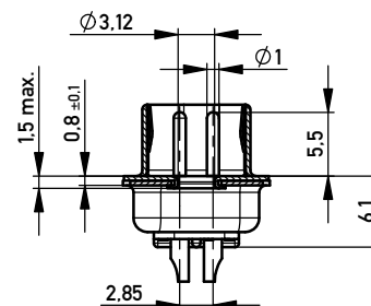
SCHNITT A-A
