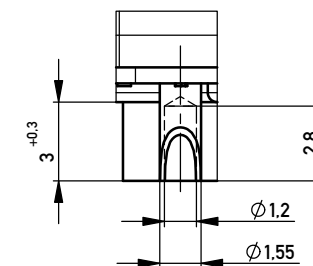
DETAIL X MAßSTAB 5 : 1
