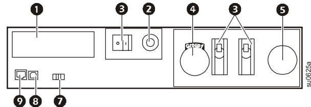
2200/3000 VA 230 V
