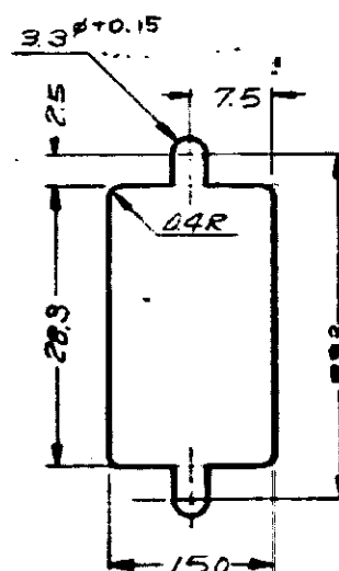
パネル切抜寸法
