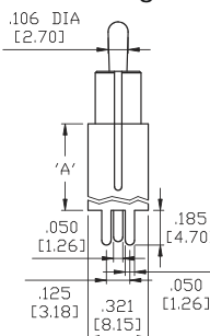
VS2-VS3 Single Pole
