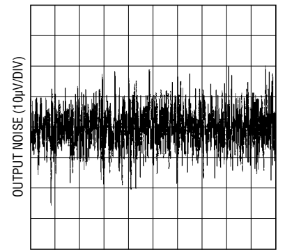
5V Output Noise 0.1\text{Hz} \leq f \leq 10\text{Hz}
