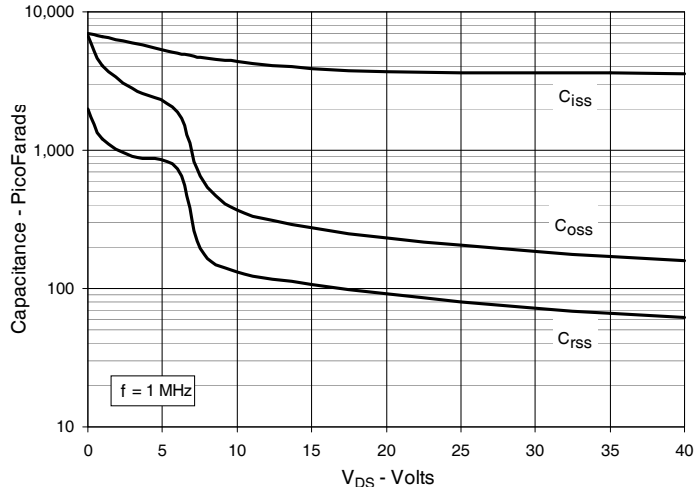
Fig. 14. Capacitance
