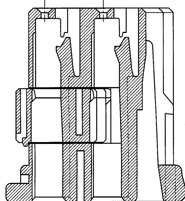
断面 C-C 断面 C-C
