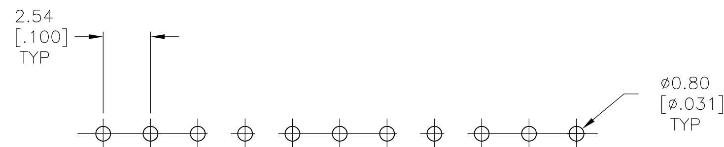
P.C.LAYOUT
