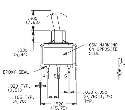
E201MD1_BE DPDT
