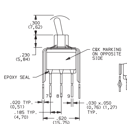
E301MD1_BE 3PDT
