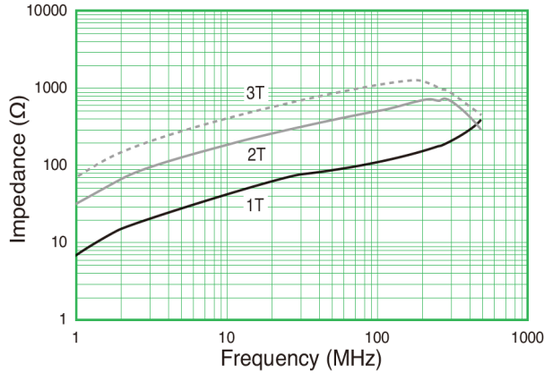
ESD-R-38C-1
