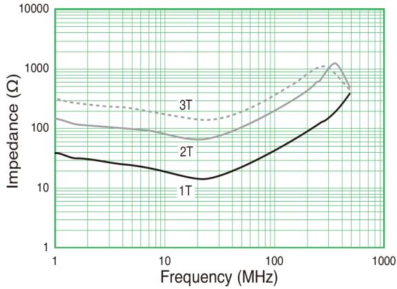
ESD-R-38
