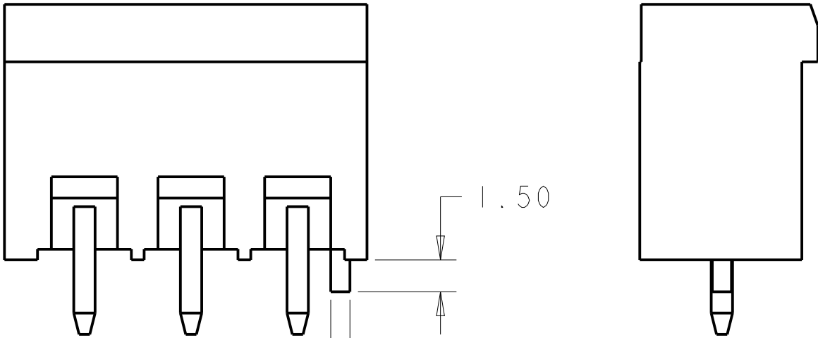
DETAIL A-A
