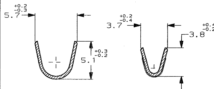
SEZIONE A-A (SECTION A-A)
