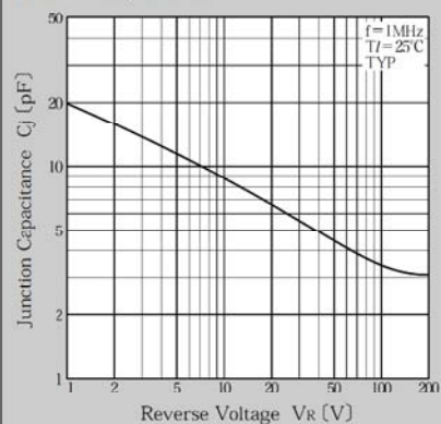
接合容量
