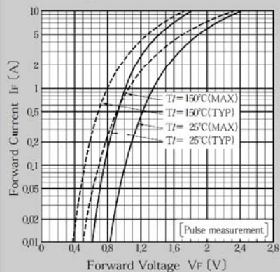
順方向特性
