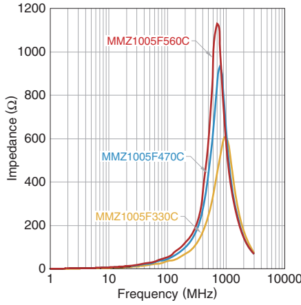
MMZ1005F 系列
