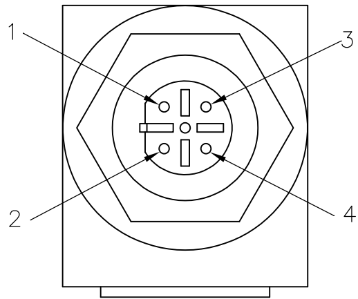
ETHERNET M12
