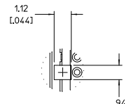
Detail C Scale 10:1 (4) PL.
