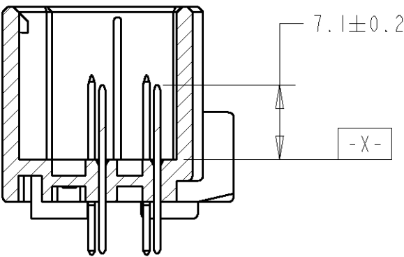
SECTION B-B SCALE 2:1
