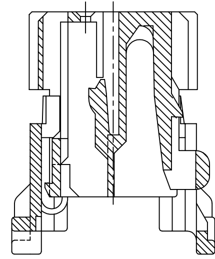
SECTION A-A (SCALE: 2.5/1)
