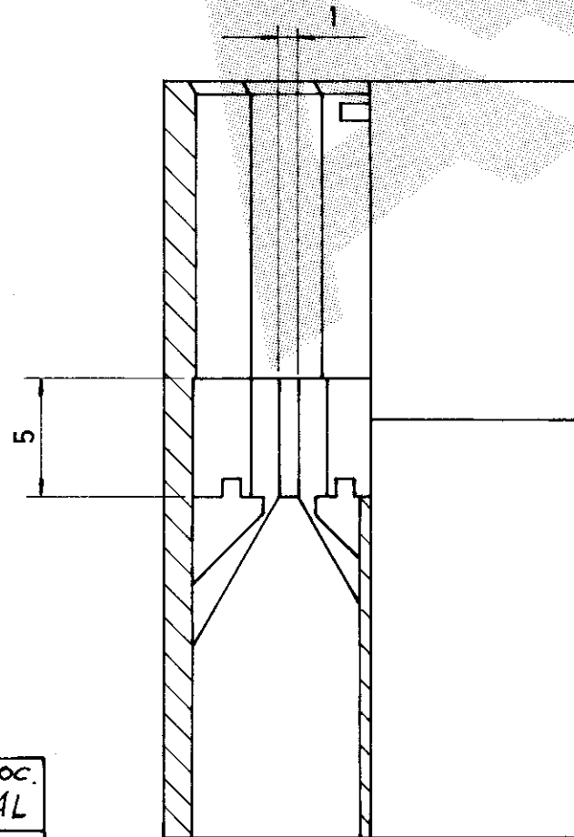
SEC. A-A
