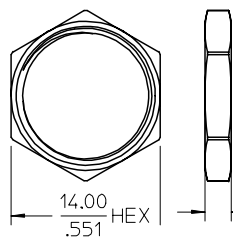
JAM NUT
