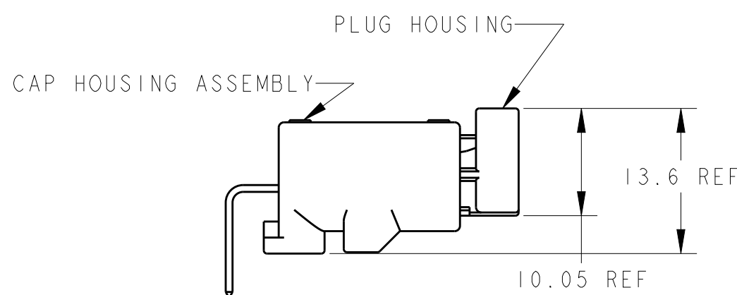
CAP HOUSING ASSEMBLY & PLUG HOUSING ENGAGEMENT VIEW キャップハウジング・アセンブリ&プラグハウジング嵌合状態図
