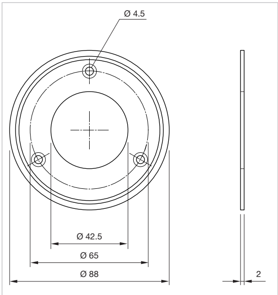
Abmessungen [mm]
