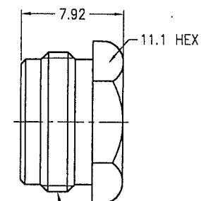
CLAMP NUT
