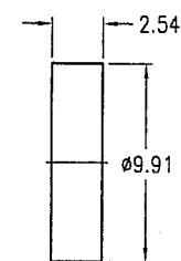
GASKET
