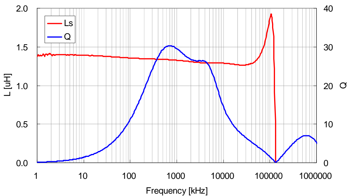
VLS3012T-1R5N1R7
