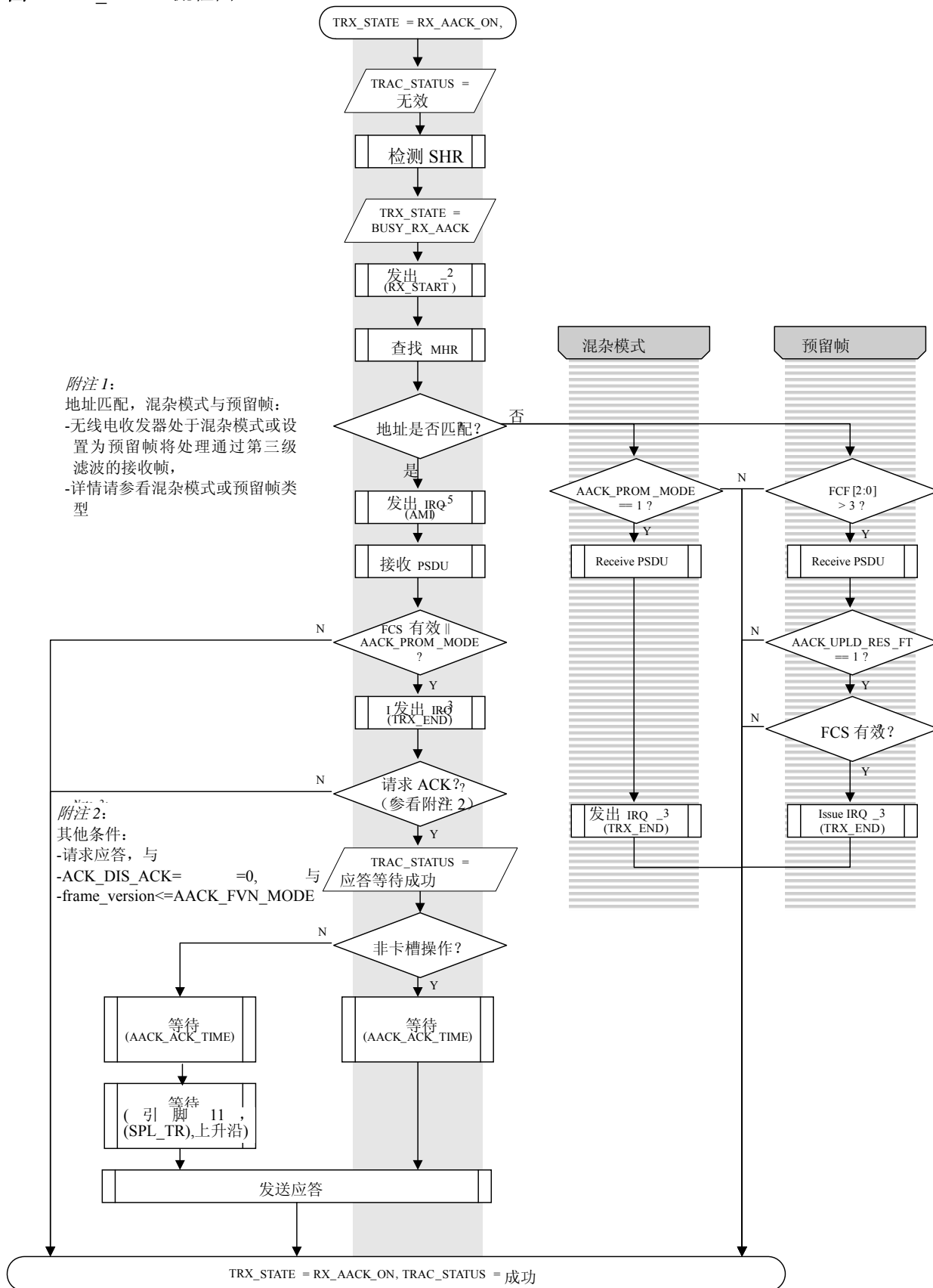
图 5-9 RX_AACK 流程图
