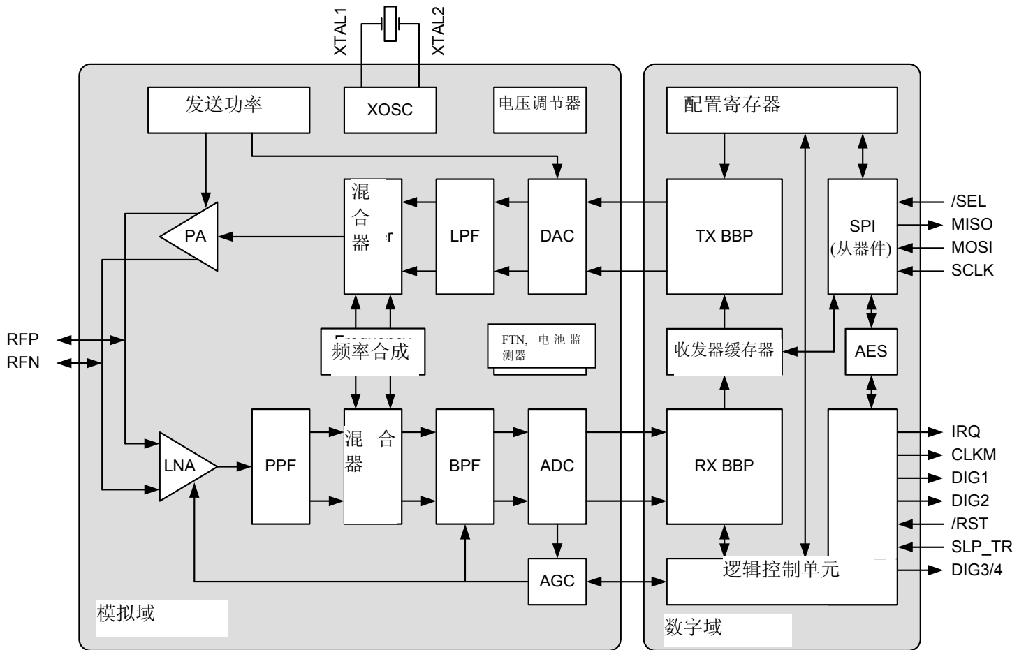
图 1-1 AT86RF212 结构图
