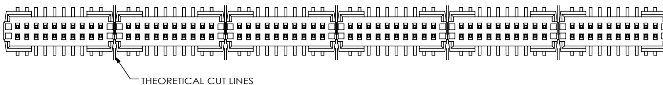
FTMH-110-XX-XX-DV-ES SHOWN (BEFORE CUT)
