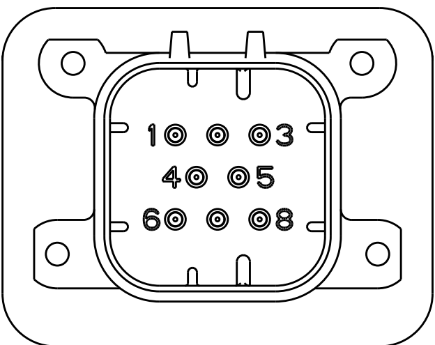
776279-1, 776279-6 & 1-776279-1 KEY LOCATION SCALE 2:1
