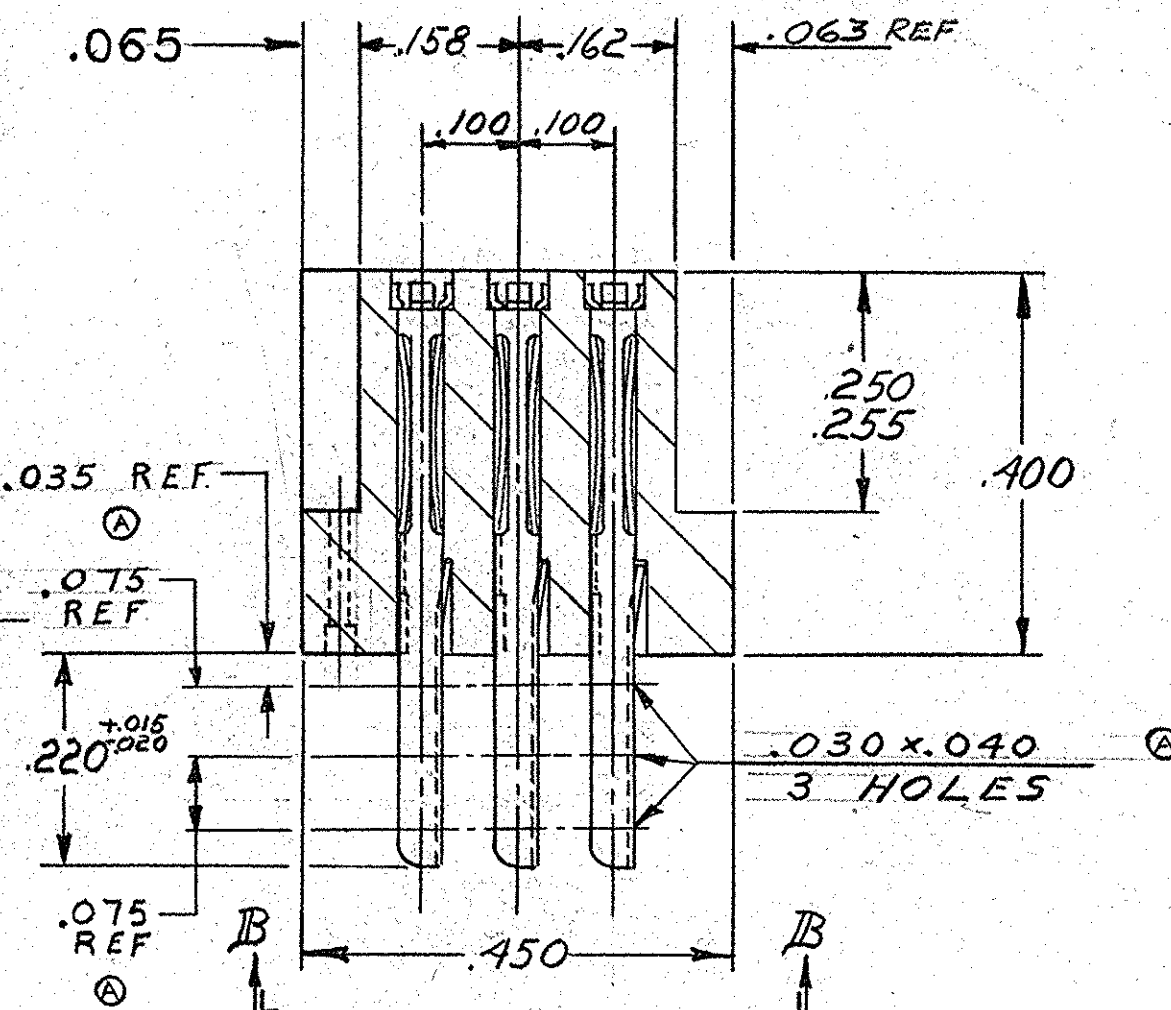
SECT A-A SCALE 5:1
