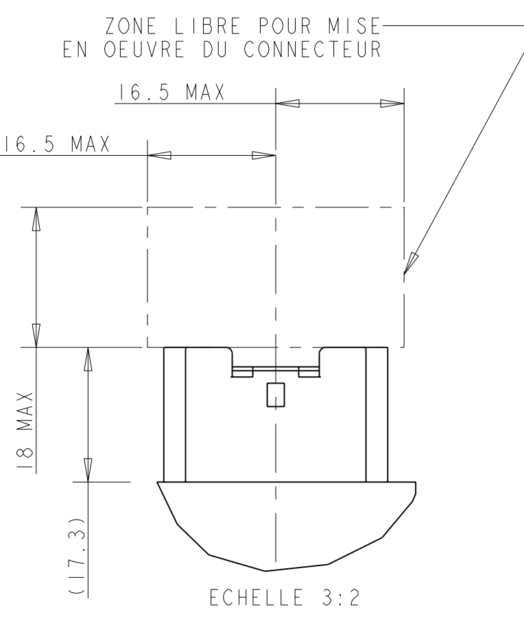
ECHELLE 3:2
