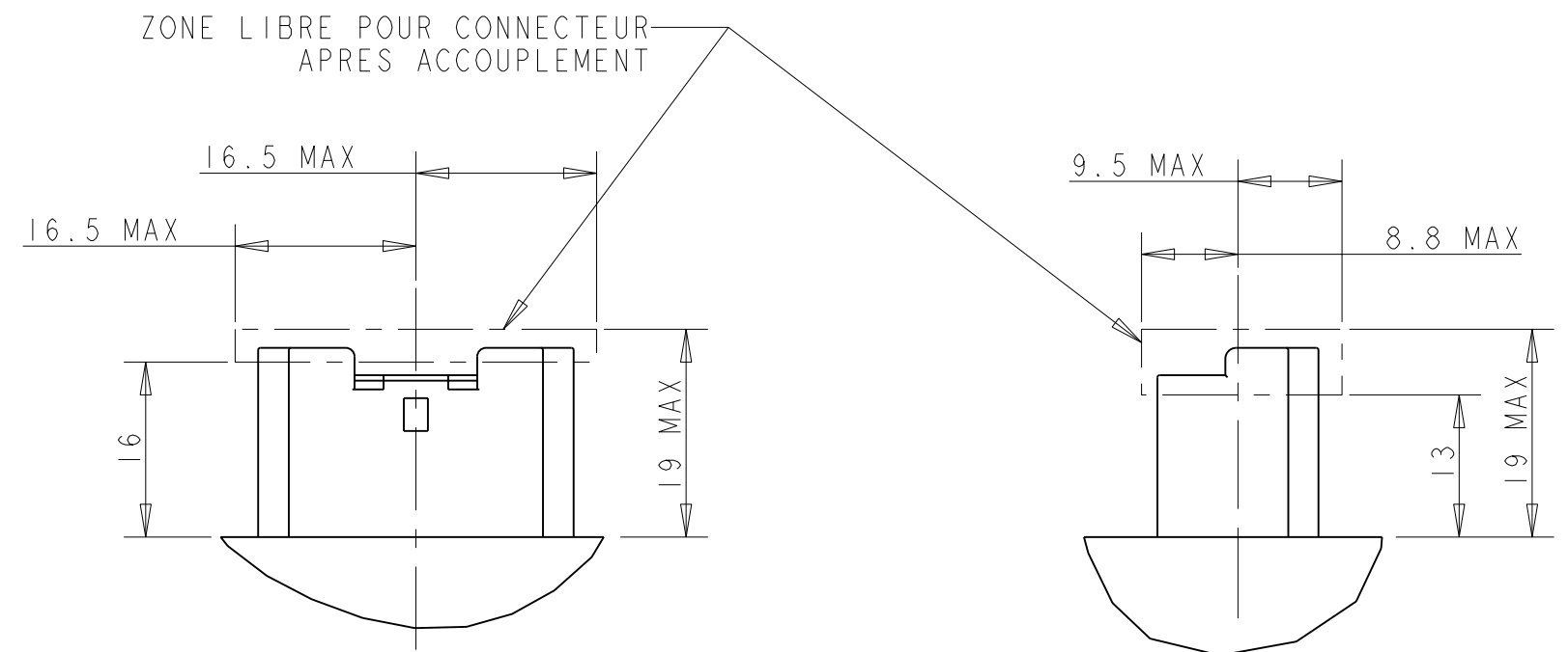
ECHELLE 3:2
