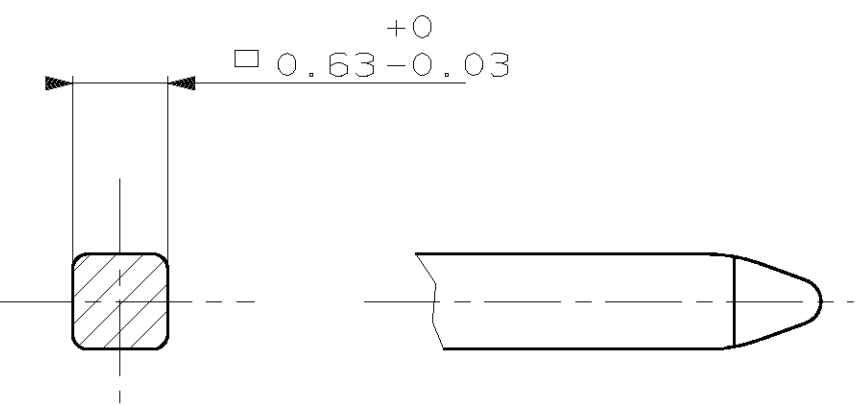
DETAIL LANGUETTES ECHELLE 20:1
